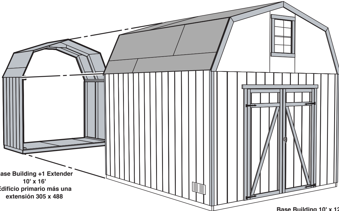
Base Building 10' x 12' Edificio primario 305 x 366
